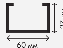
Профиль потолочный (стоечный) ПП 60x27 мм
