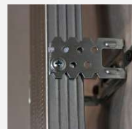
Крепление подвесов к ПП с помощью саморезов с прессшайбой
