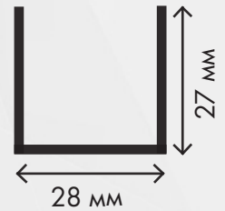
Направляющая горизонтальная НПП 28x27 мм
